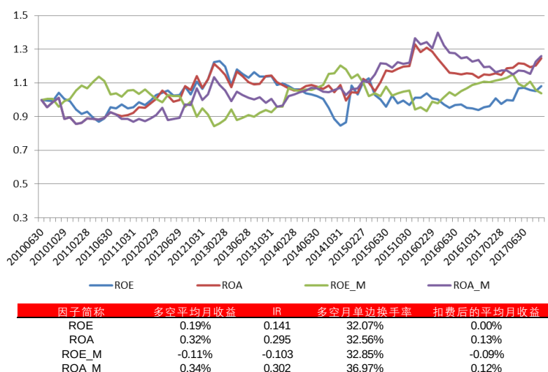
图 6：盈利能力因子多空净值和表现
